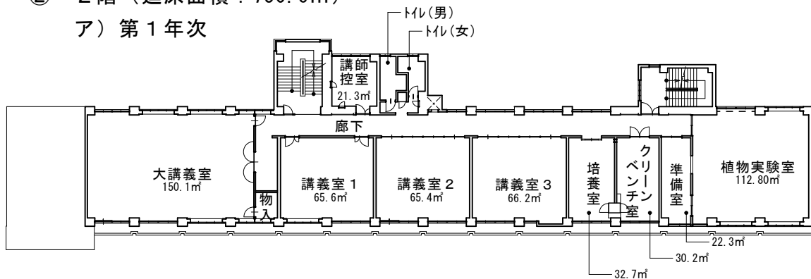
< 2階平面図（第1年次） >
