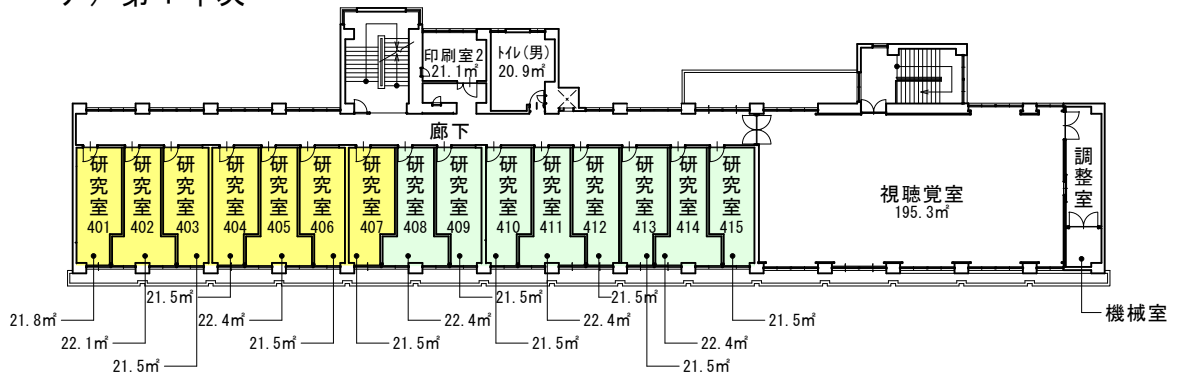
< 4階平面図（第1年次） >
