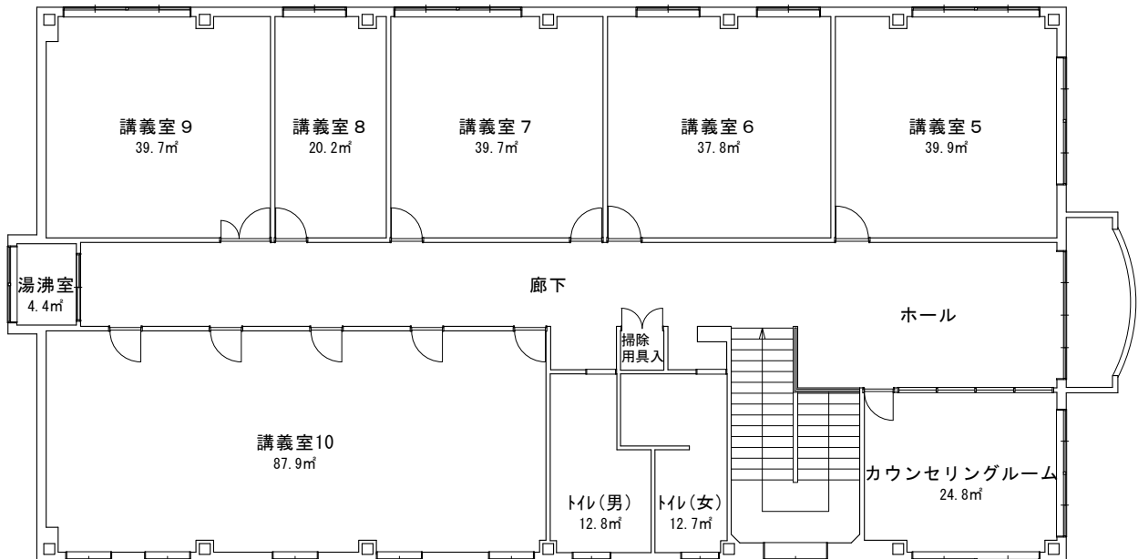
< 2階平面図 >
