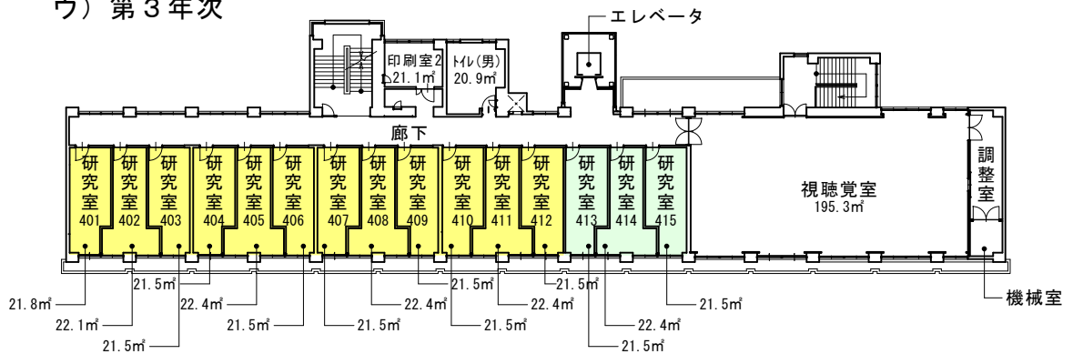
< 4階平面図（第3年次～） >
