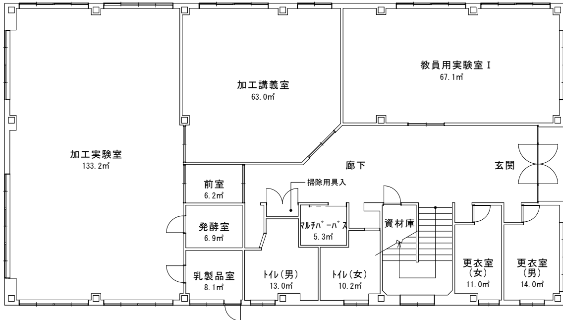
< 1階平面図 >
