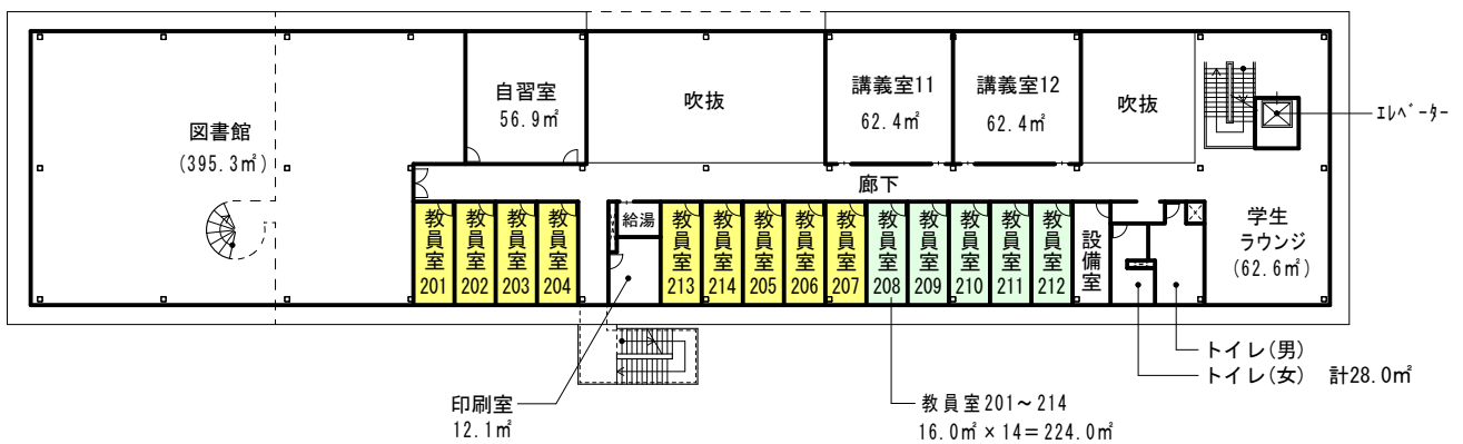
< 2階平面図 (第2年次) >
