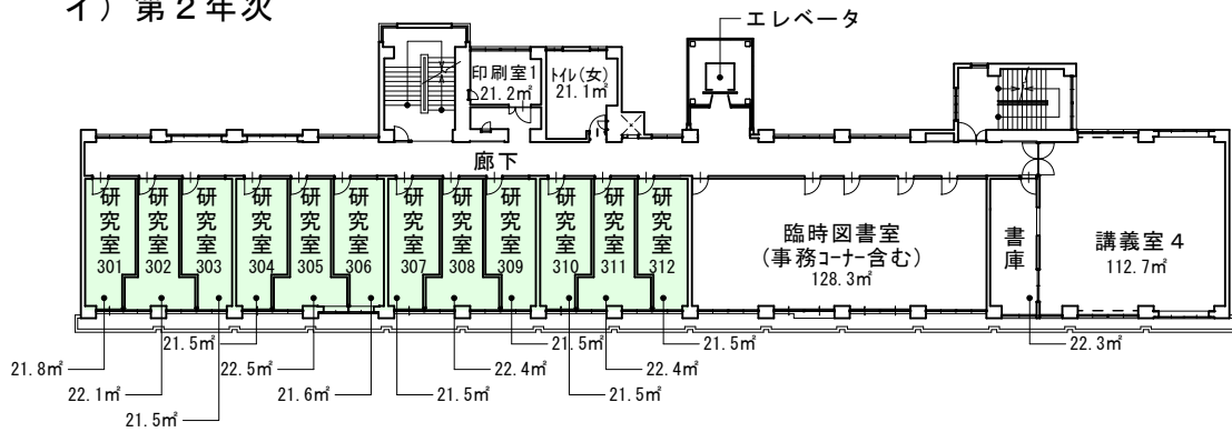
< 3階平面図（第2年次） >
