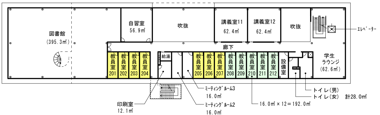
< 2階平面図 (第3年次～) >
