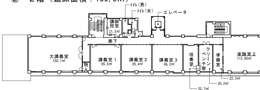
< 2階平面図 >
